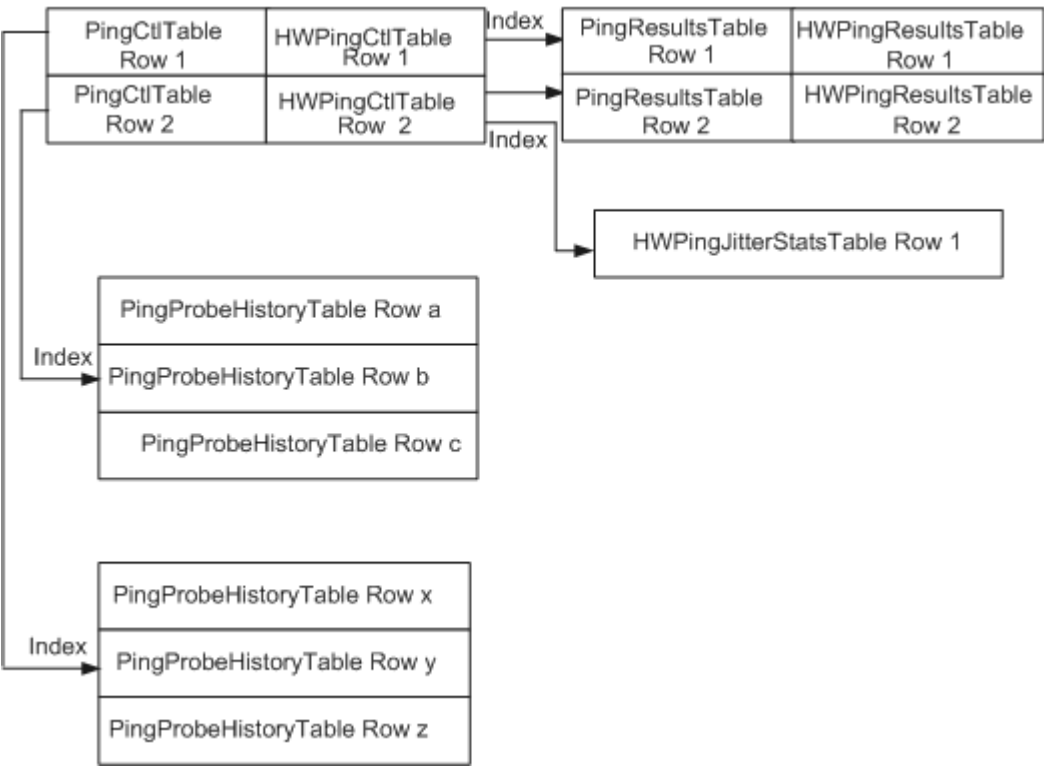
图 7-1 DISMAN-PING-MIB 表间关系图
